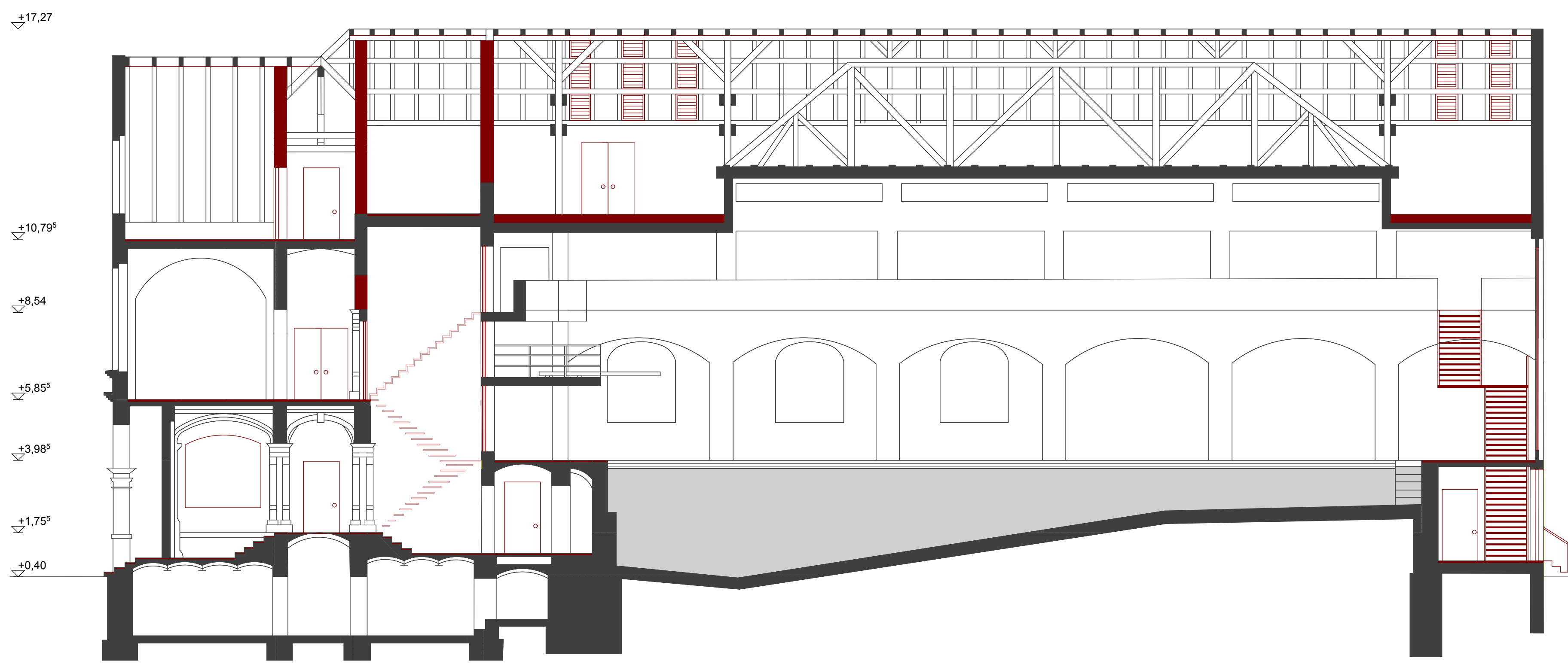
SCHNITT LÄNGS M 1:100
