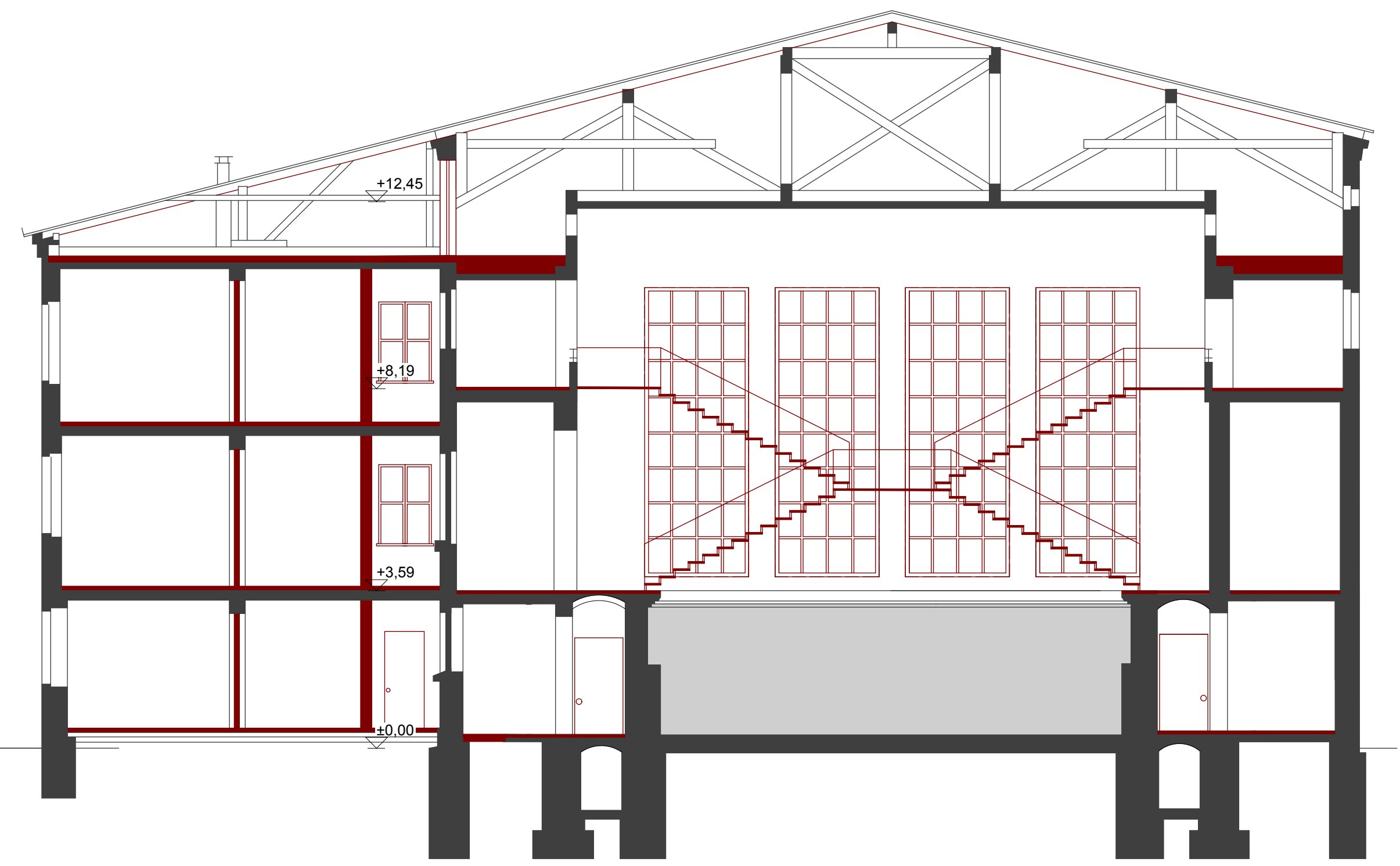
SCHNITT QUER M 1:100
