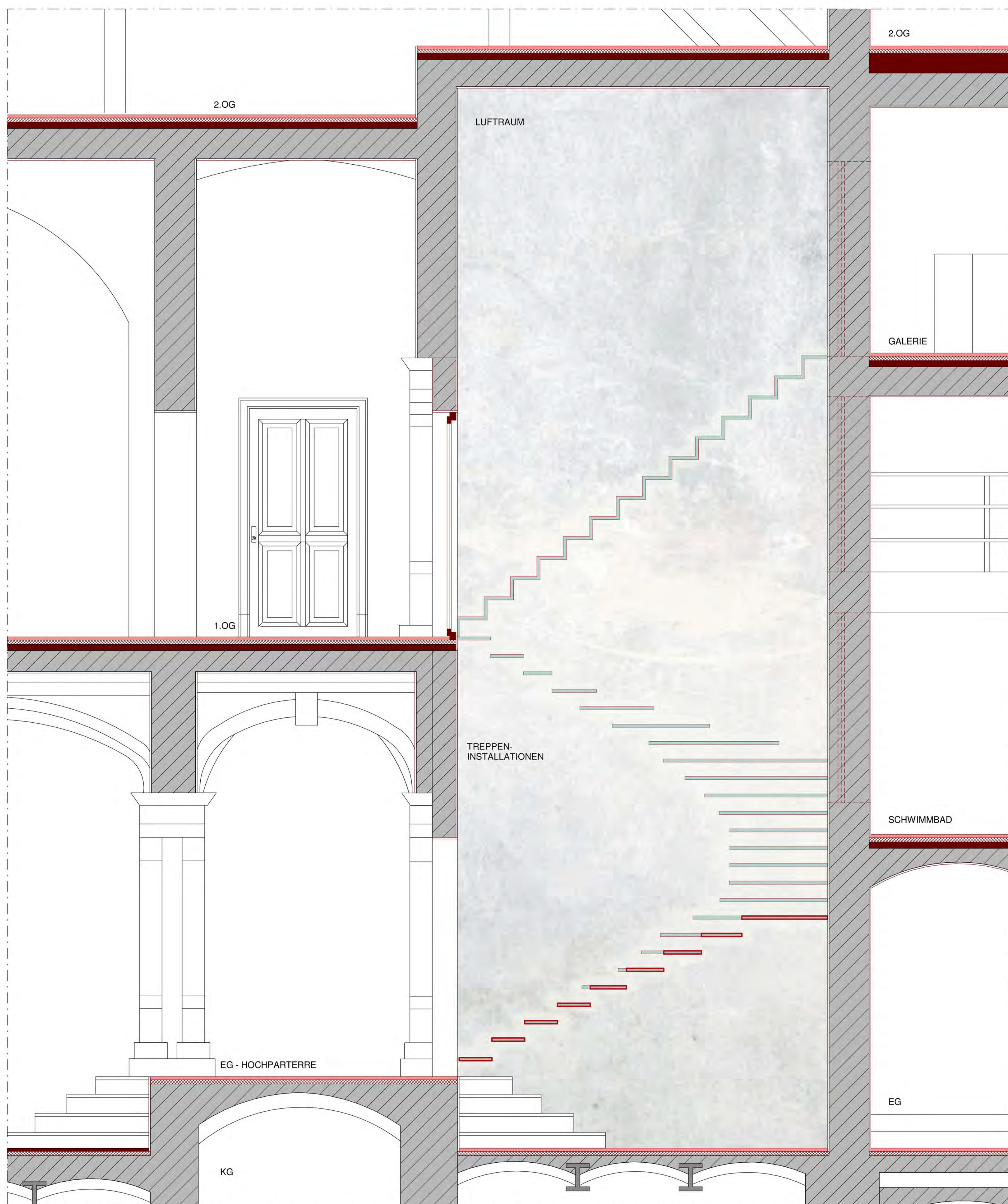
DETAILSCHNITT M 1:20
