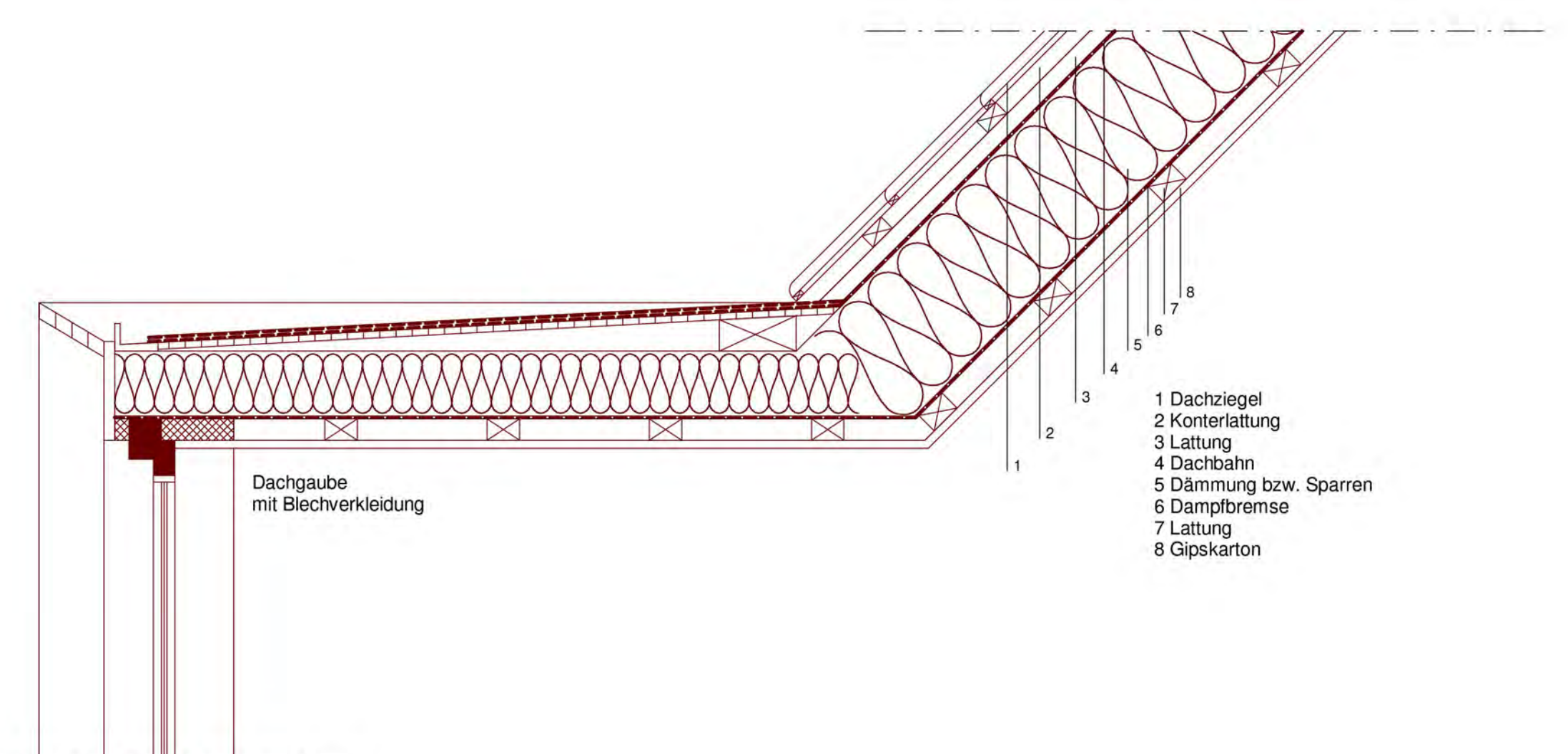
DACHGAUBE M 1:10
